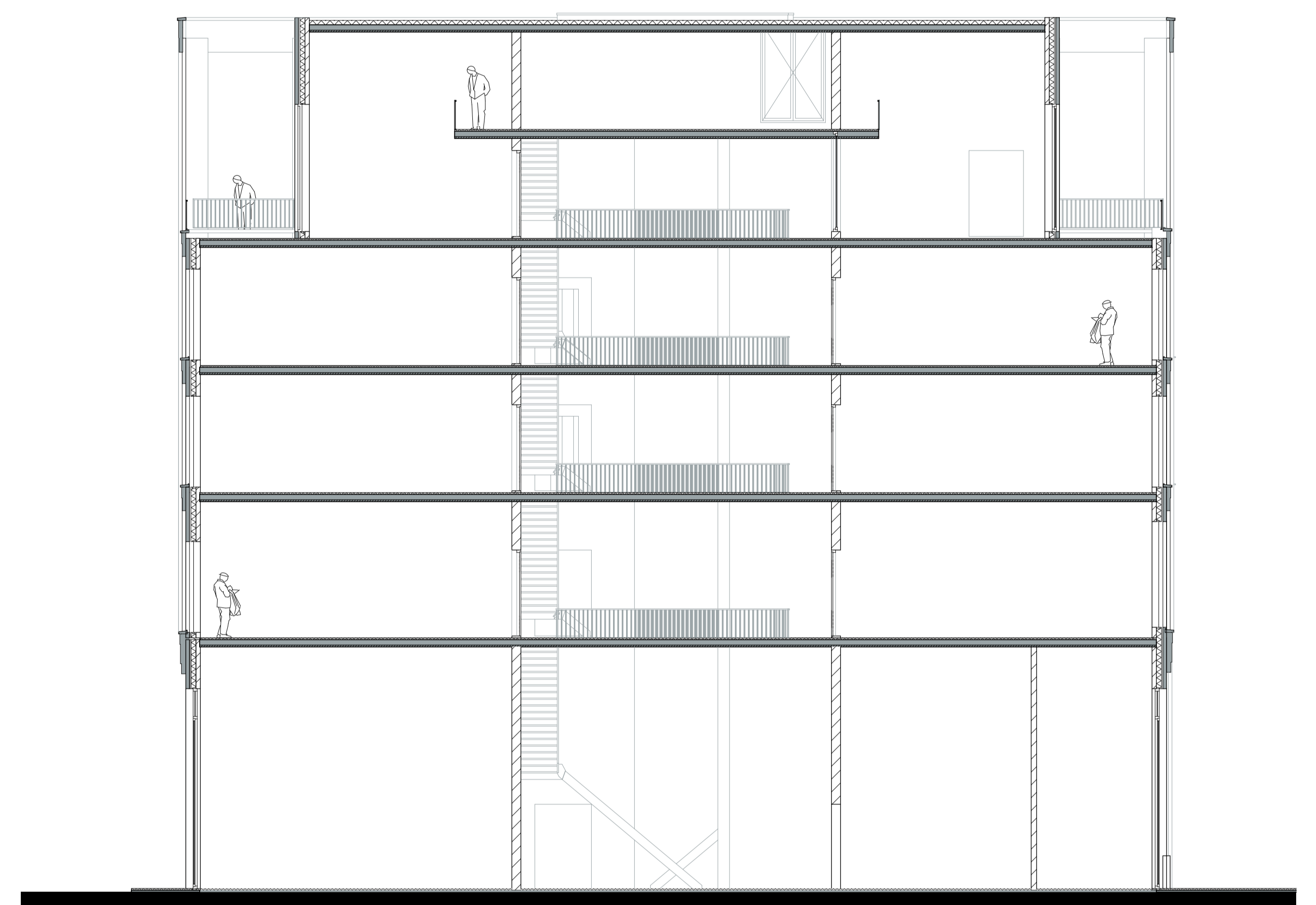
SECTION A-A
