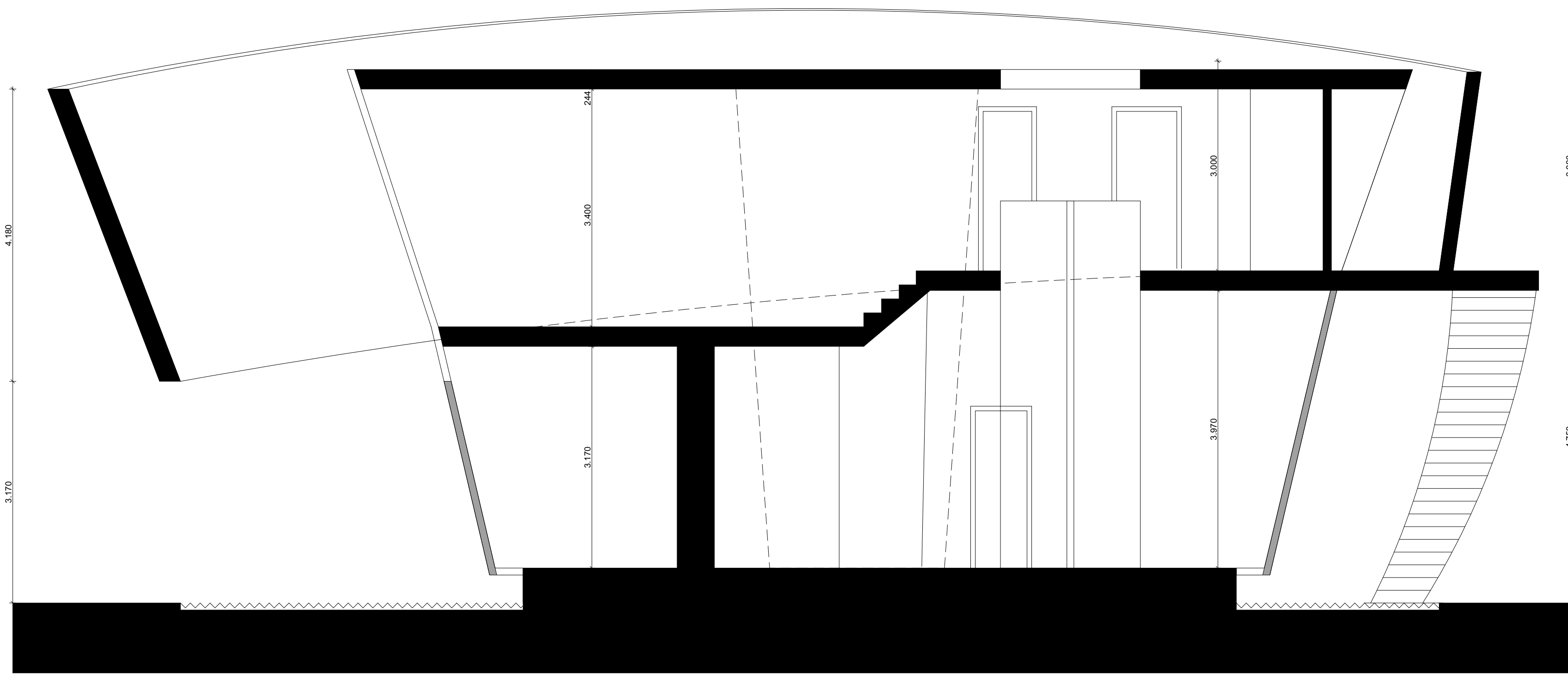
DOORSNEDE B-B
