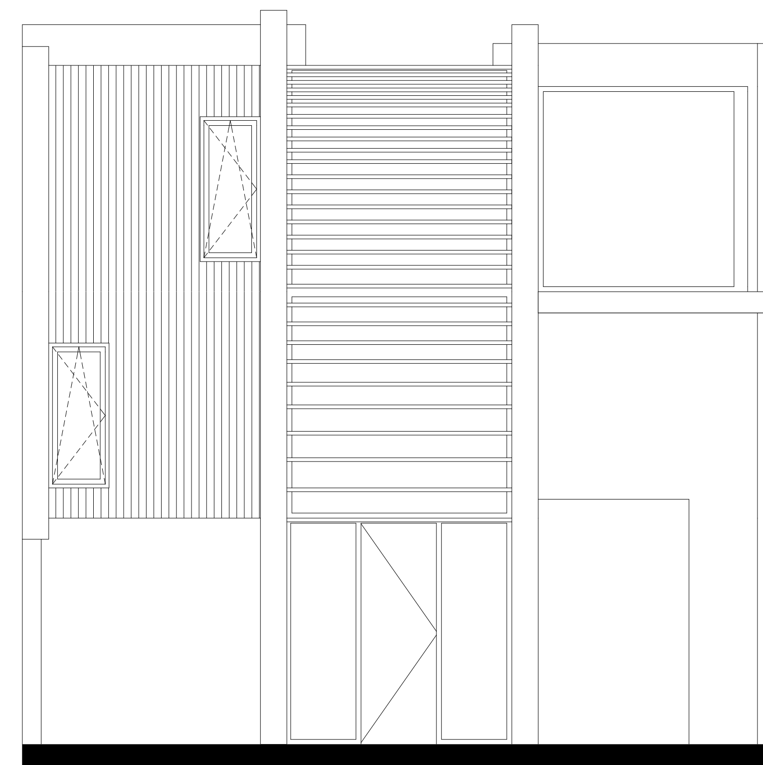
VOORGEVEL (OOST)
