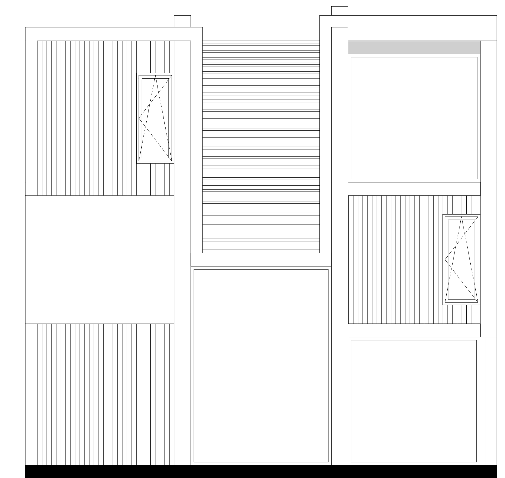
ACHTERGEVEL (WEST)
