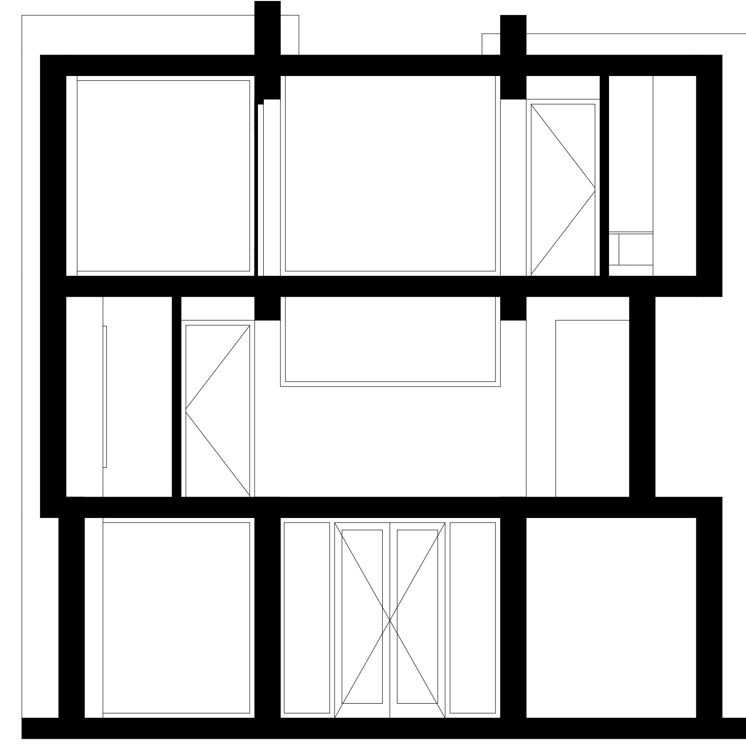
DOORSNEDE B-B
