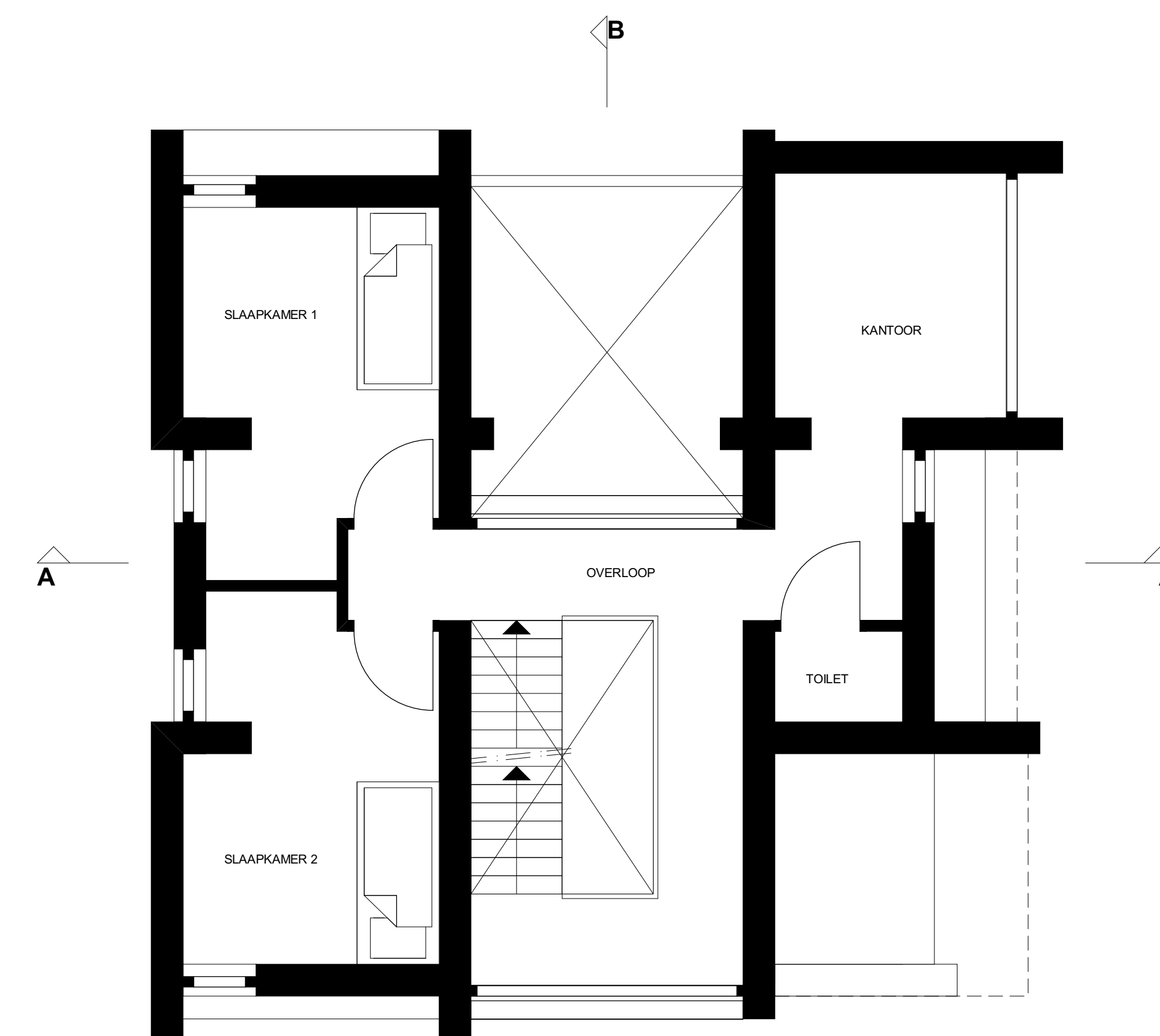
1e VERDIEPING
