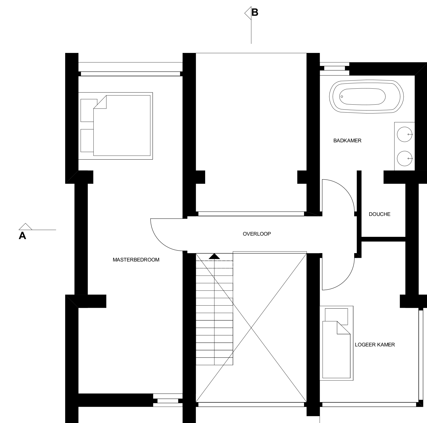
2e VERDIEPING
