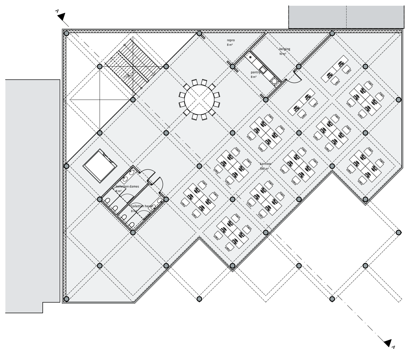
2e verdieping, 1:200
