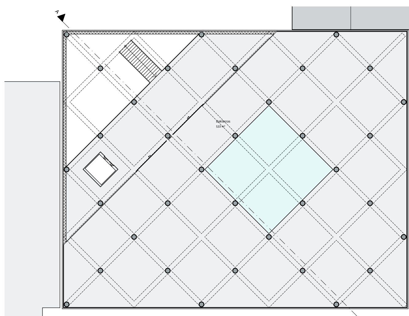
4e verdieping, 1:200
