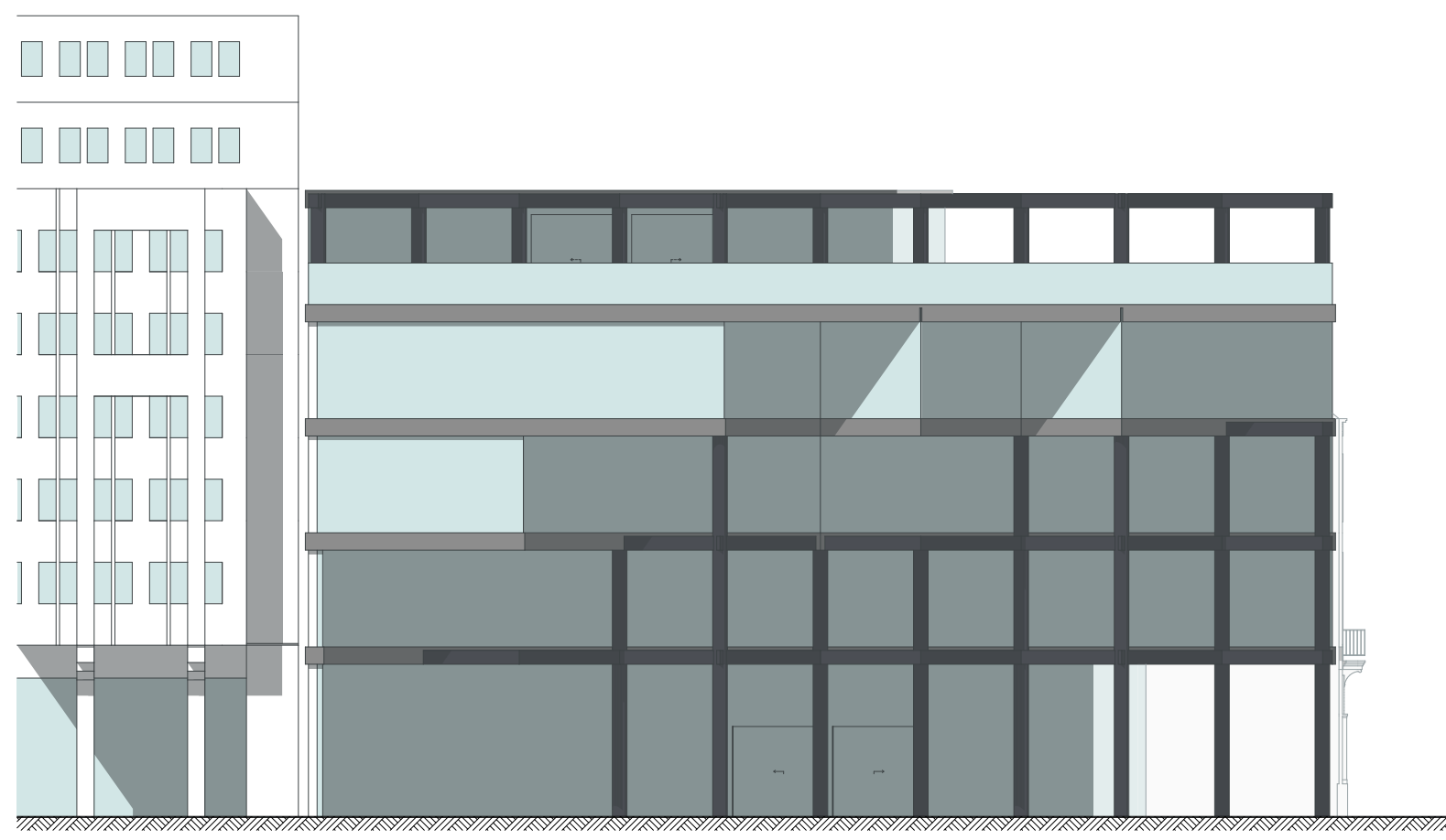
Zuidgevel, 1:200
