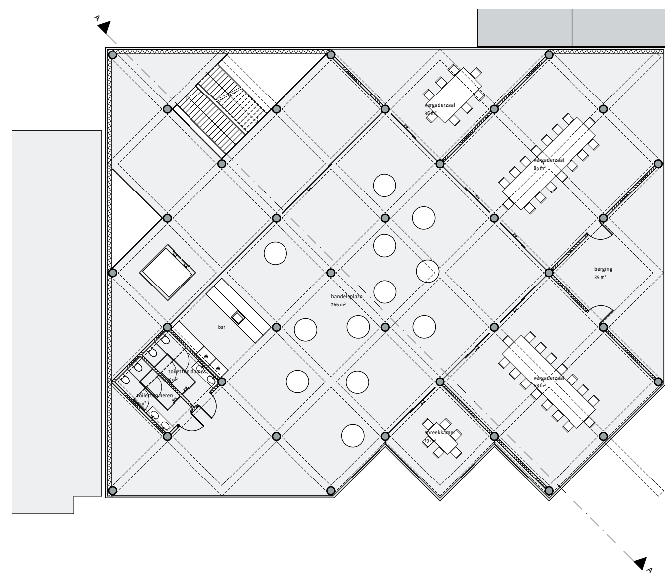
3e verdieping, 1:200
