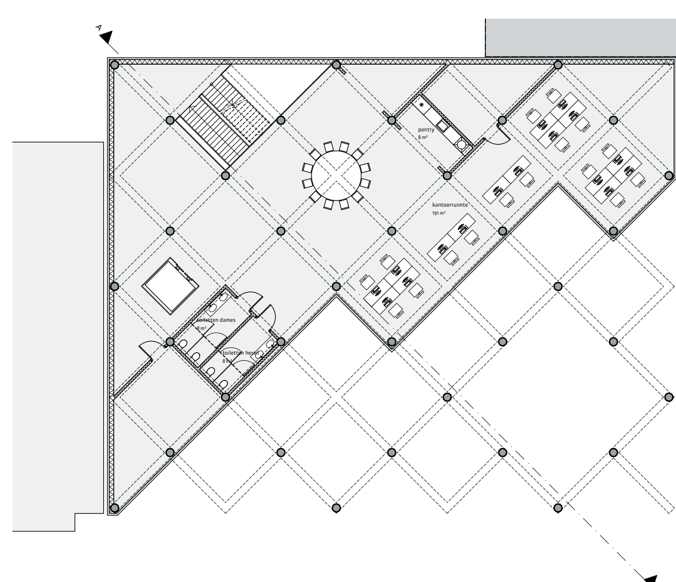
1e verdieping, 1:200
