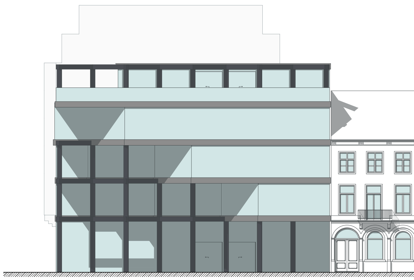
Oostgevel 1:200
