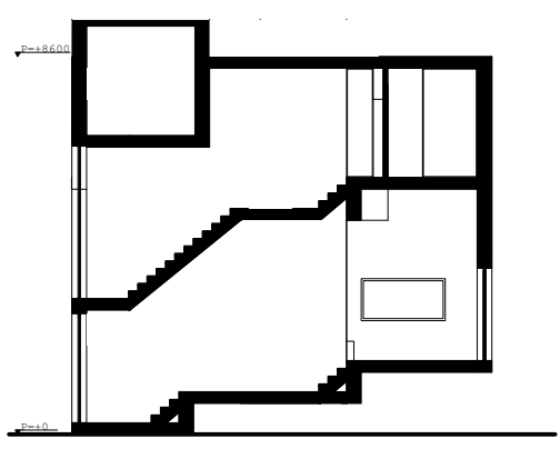
Doorsnede A-A'
