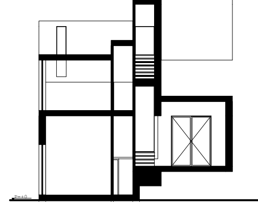
Doorsnede B-B'
