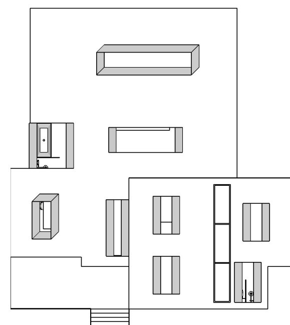
Doorsnede B-B'
