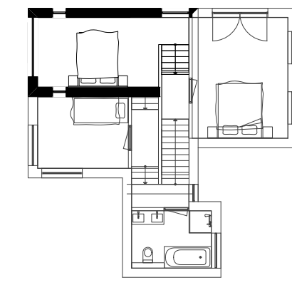
Tweede verdieping
