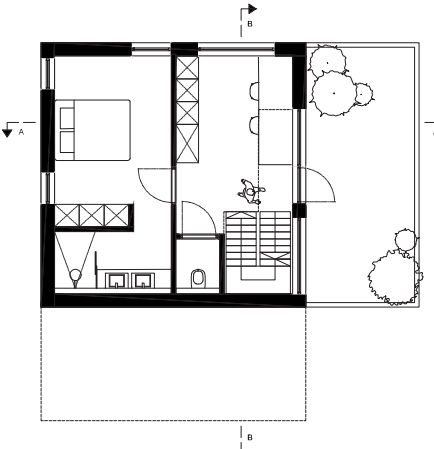
1e verdiepingvloer
