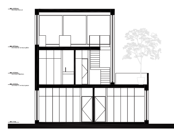
Doorsnede A-A
