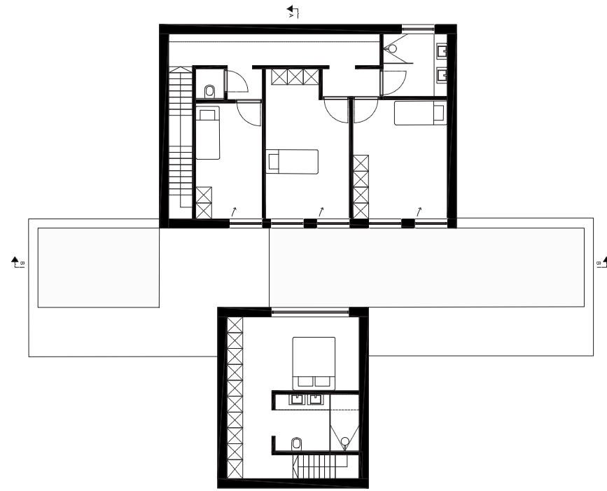
1e verdiepingvloer
