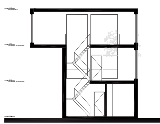
Doorsnede B-B
