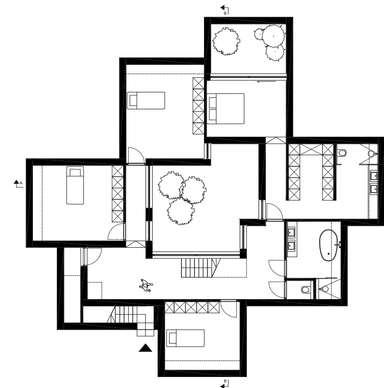
Begane grondvloer
