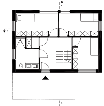
Begane grondvloer
