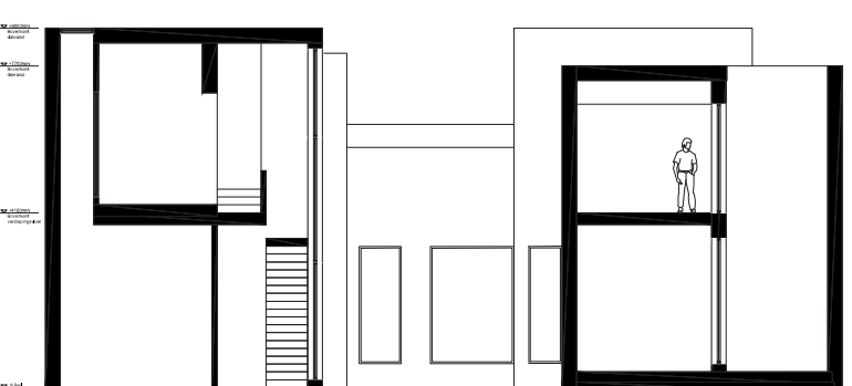
Doorsnede B-B
