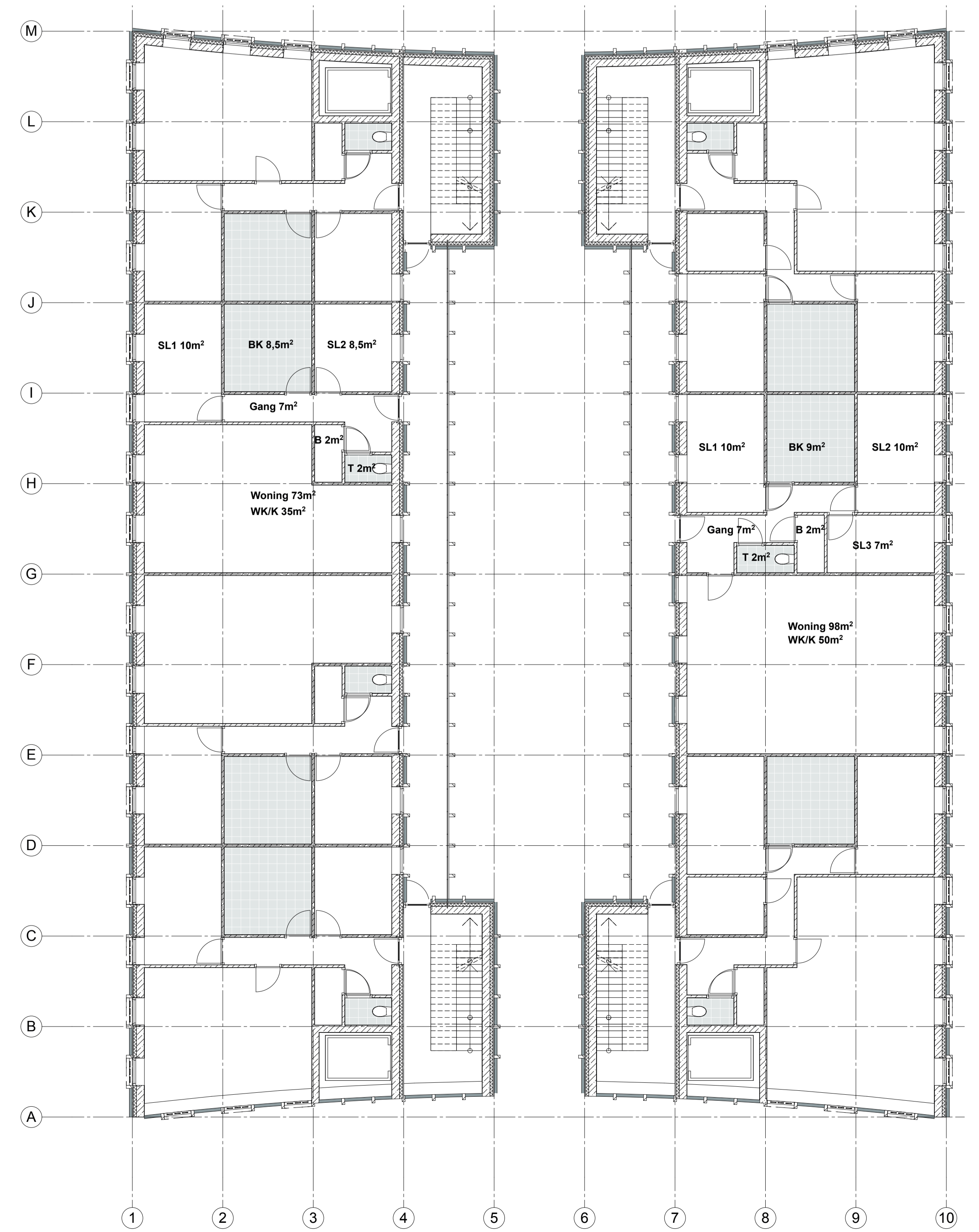
1:100 Plattegrond 1 e t/m 5 e
