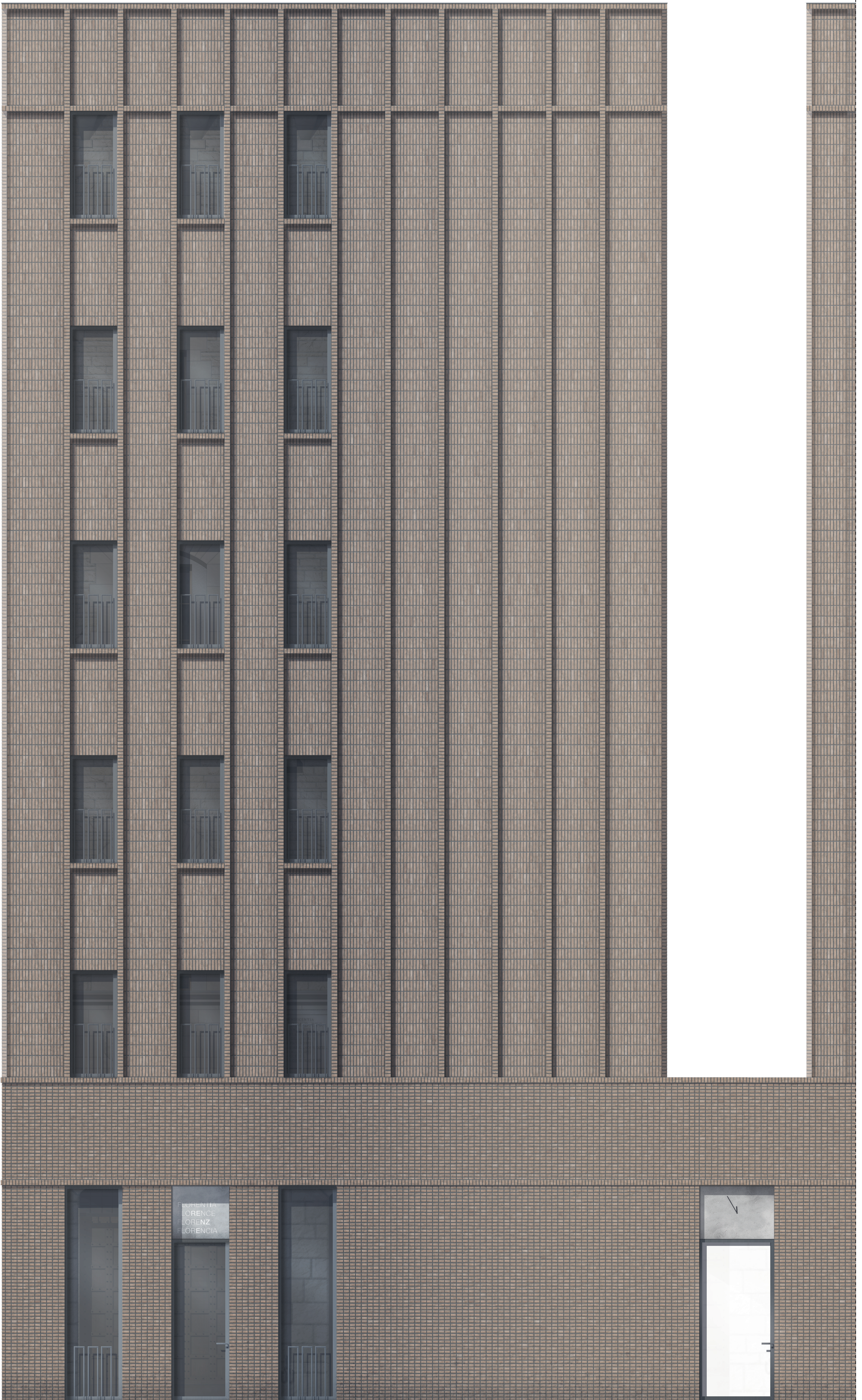
1:20 Voorgevel
